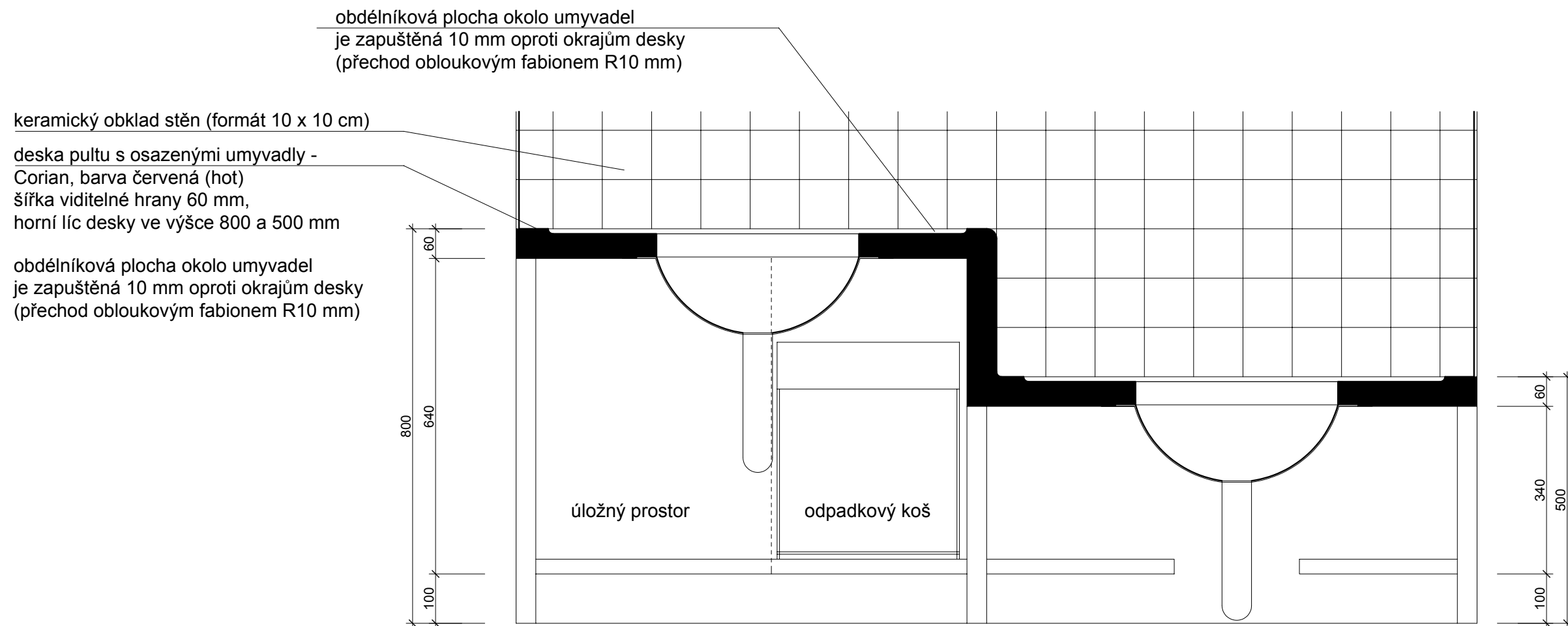
Řez A - A 1:10
