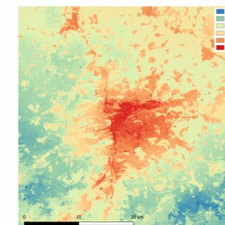
IFS-NEMO SSP3-7.0 2031-2040
